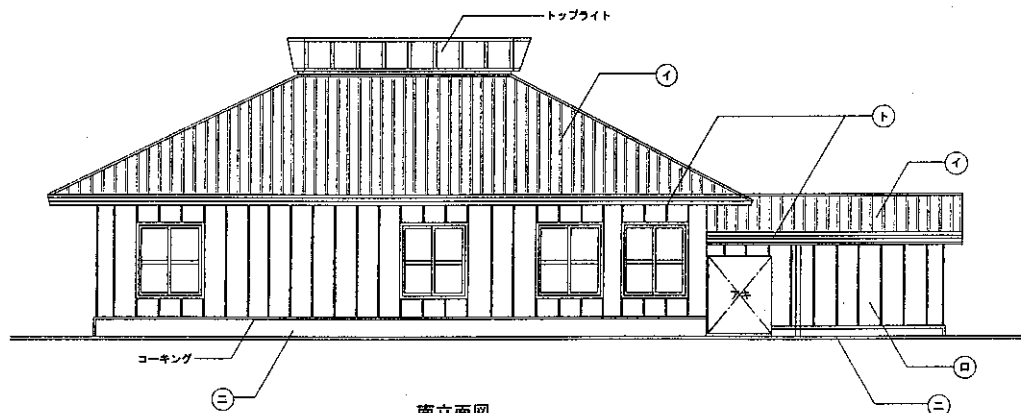
南立面図
