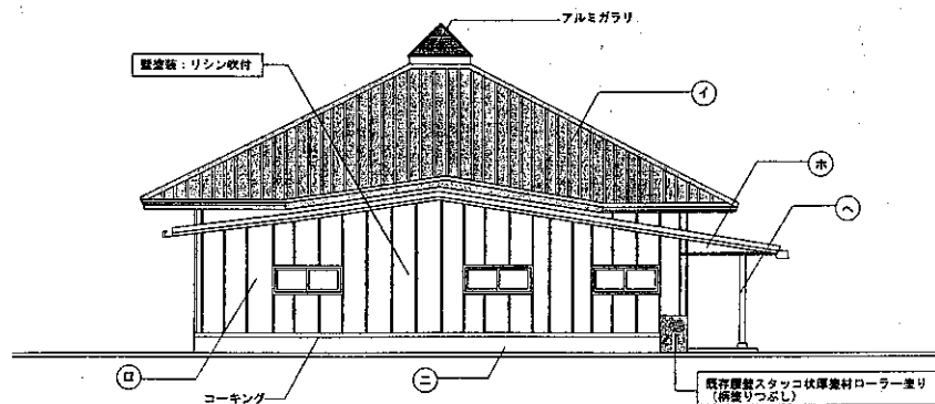
東立面図
