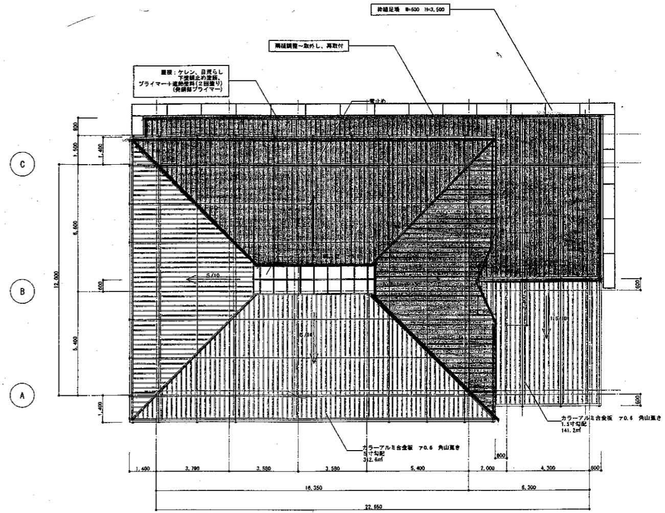
屋根伏図
