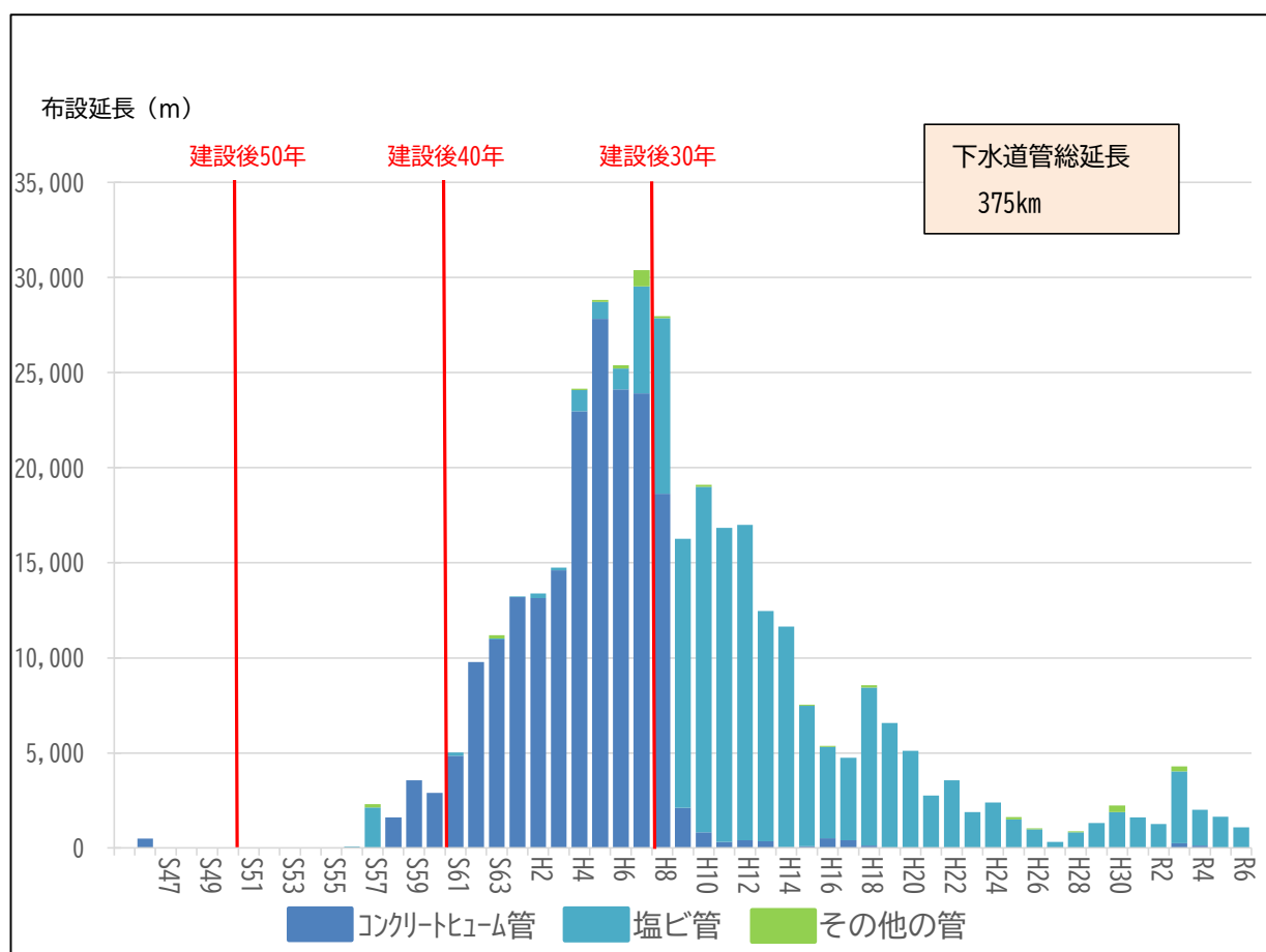
【図- 36 年度別下水道整備延長】
