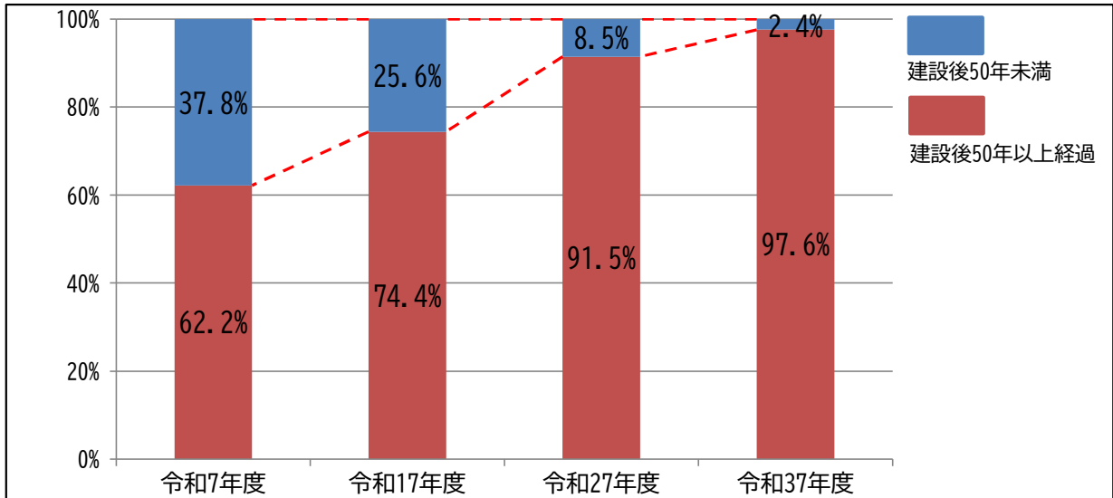
【図- 33 更新時期を迎える車道橋の割合】
