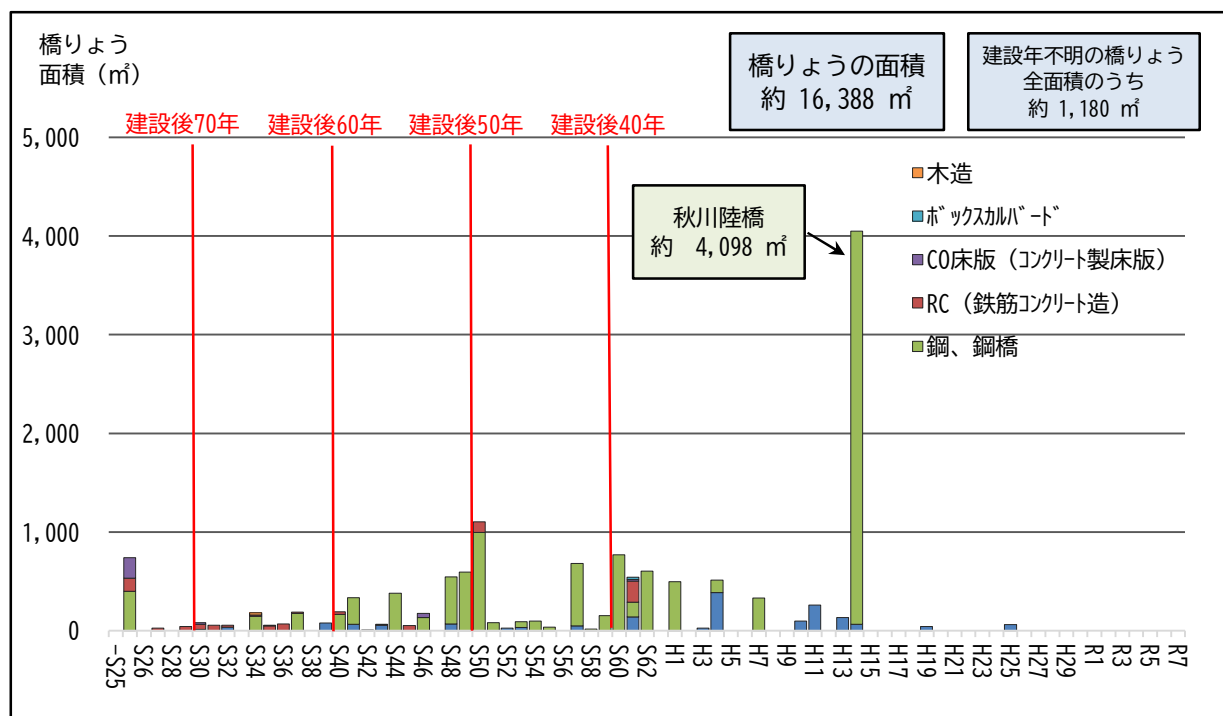
【図-32 年別橋りょう新設整備面積(構造別)】
