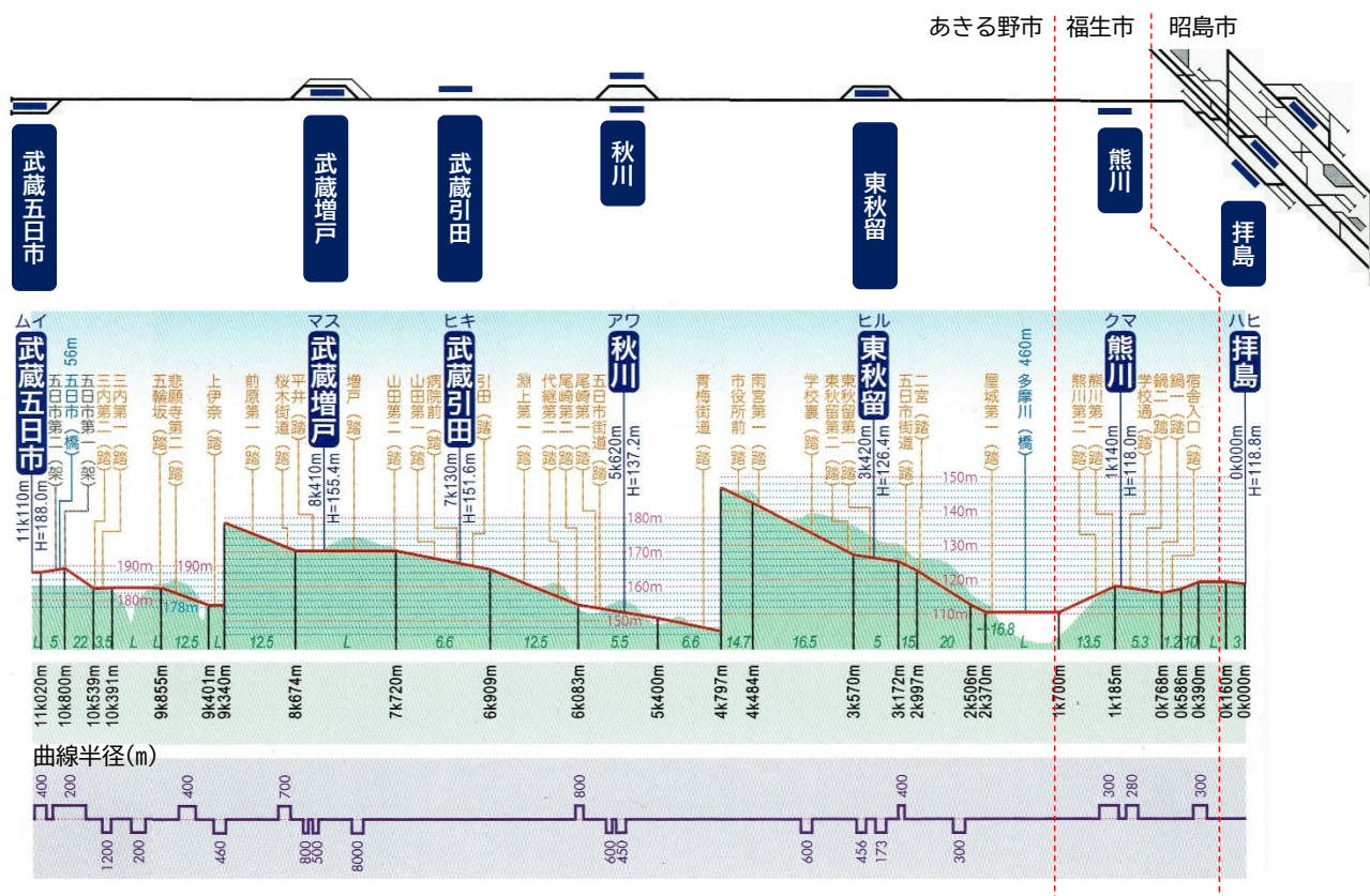
図 2-29 JR 五日市線配線略図（上）及び縦断面図（下）
